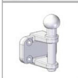
610-MC11001 Kugel-Maul-Lupplung 4-Loch Flansch 83x56x11
